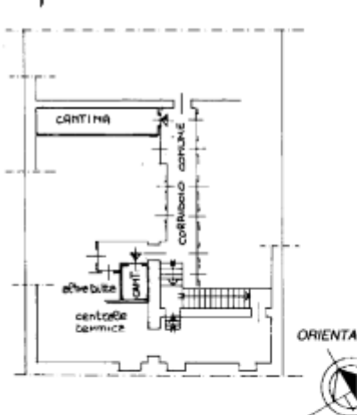
PIANTA PIANO INTERRATO H = 3.00 mt.
